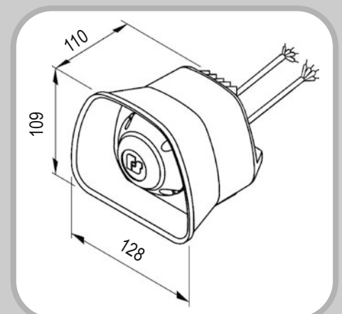
SCS1000-D Siren dimensions in mm.
